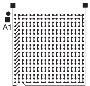
CBGA361
